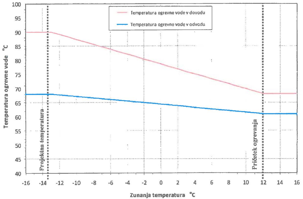
Priloga 2: Temperaturni diagram za zunanjo projektno temperaturo – 13 °C
